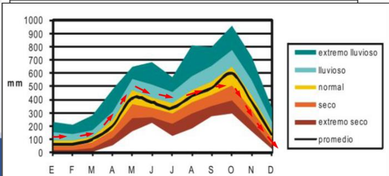
Precipitación promedio en comparación con cinco rangos de variabilidad climática Pacífico Central
